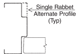
Jamb or Head
